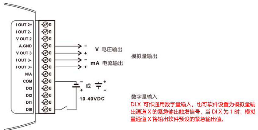
SP-4024 模拟量输入、数字量输出接线图 b
